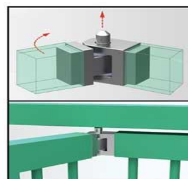
Particolare Art. CB PERNO a scomparsa in INOX
